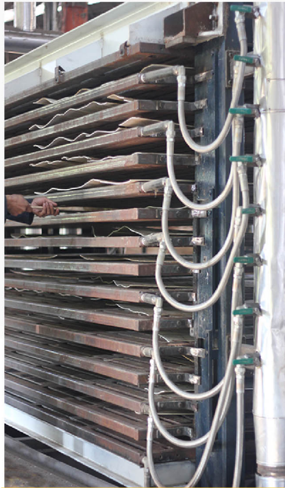
PRESS DRYER
